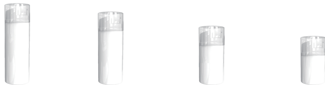
C : 100ml D : 45mm H : 138mm M : AS.PP C : 80ml D : 45mm H : 120mm M : AS.PP C : 50ml D : 45mm H : 98mm M : AS.PP C : 30ml D : 45mm H : 82mm M : AS.PP
